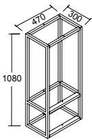
Kit struttura Structure kit
