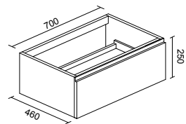
Base sospesa con 1 cassetto Wall cabinet with 1 drawer
