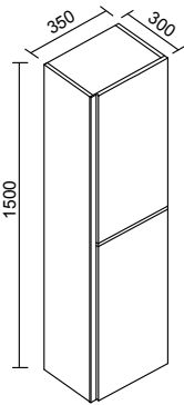
Colonna sospesa con 2 ante Wall high cabinet with 2 doors
