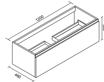
Base sospesa porta lavabo con 1 cassetto Wall wash-stand with 1 drawer
