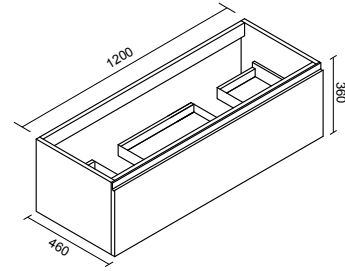
Base sospesa porta lavabo doppia vasca con 1 cassetto Double sink wall wash-stand with 1 drawer
