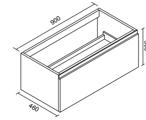
Base sospesa con 1 cassetto Wall cabinet with 1 drawer
