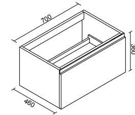
Base sospesa con 1 cassetto Wall cabinet with 1 drawer
